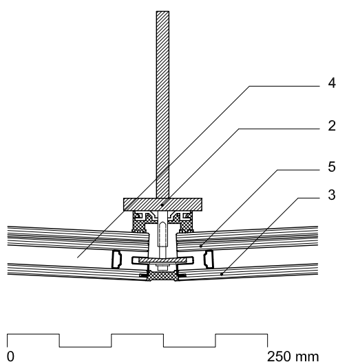
Dettaglio Sezione orizzontale
